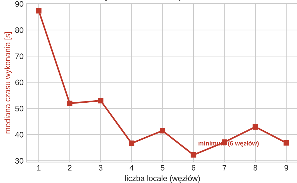
Czas wykonania nie maleje monotonicznie
