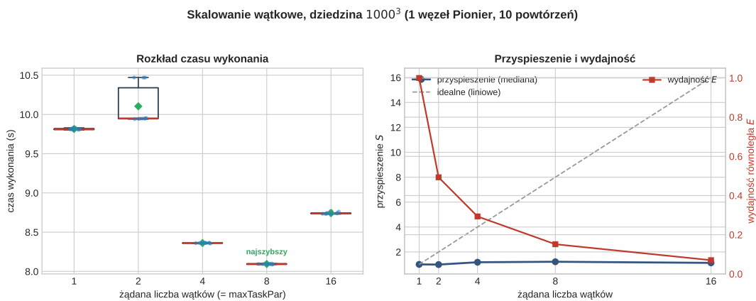
Rysunek 5.1: Skalowanie wątkowe dla dziedziny 1000^3 na węźle Pionier. Lewy panel: rozkład czasu wykonania w postaci wykresu pudełkowego w funkcji liczby wątków. Prawy panel: zmierzone przyspieszenie na tle przyspieszenia idealnego oraz wydajność E .
