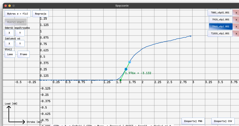
Rysunek 5.16: Wykres siły w funkcji przemieszczenia w trakcie operacji
