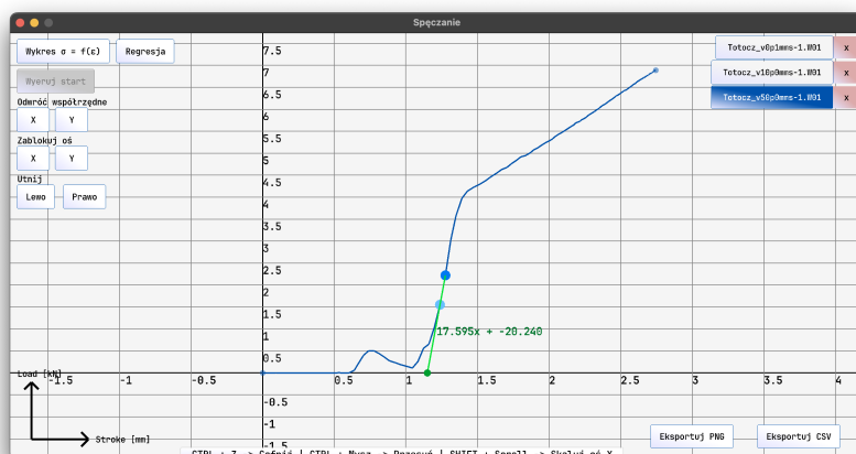
Rysunek 5.11: Wykres siły w funkcji przemieszczenia w trakcie operacji
