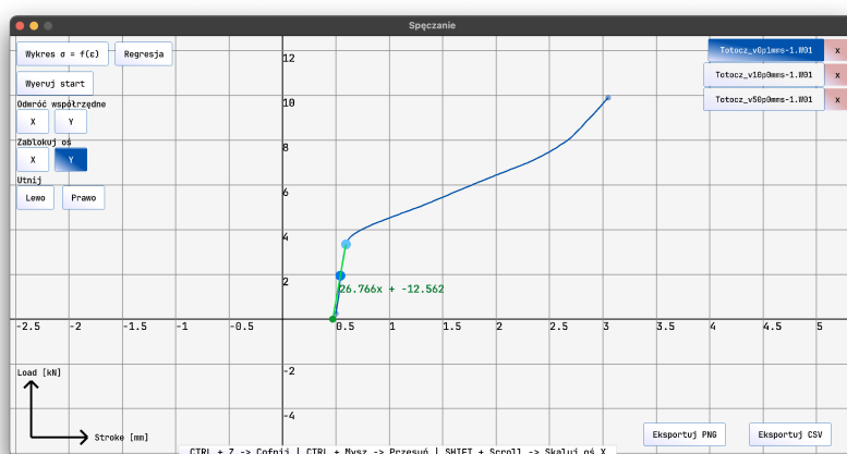
Rysunek 5.7: Wykres siły w funkcji przemieszczenia w trakcie operacji
