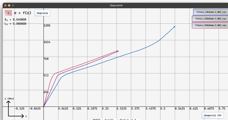
Rysunek 5.12: Wykres naprężenie-odkształcenie dla próbek CuSn6 spęczanych w temperaturze otoczenia
