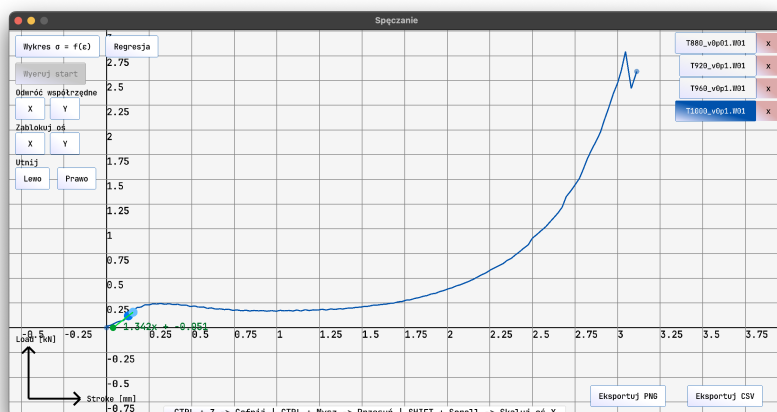
Rysunek 5.18: Wykres siły w funkcji przemieszczenia w trakcie operacji
