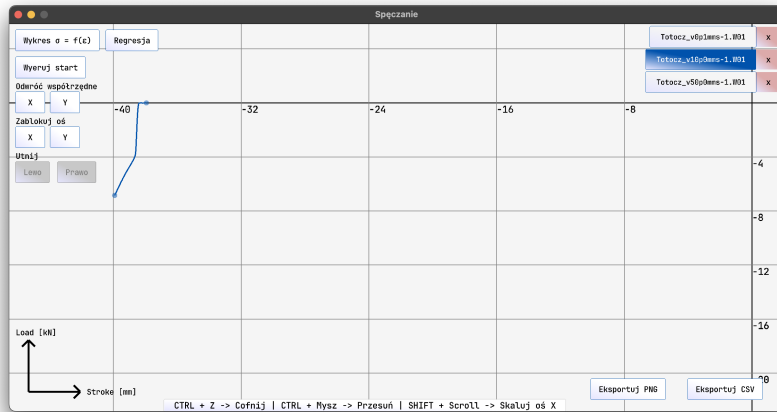
Rysunek 5.8: Wykres siły w funkcji przemieszczenia
