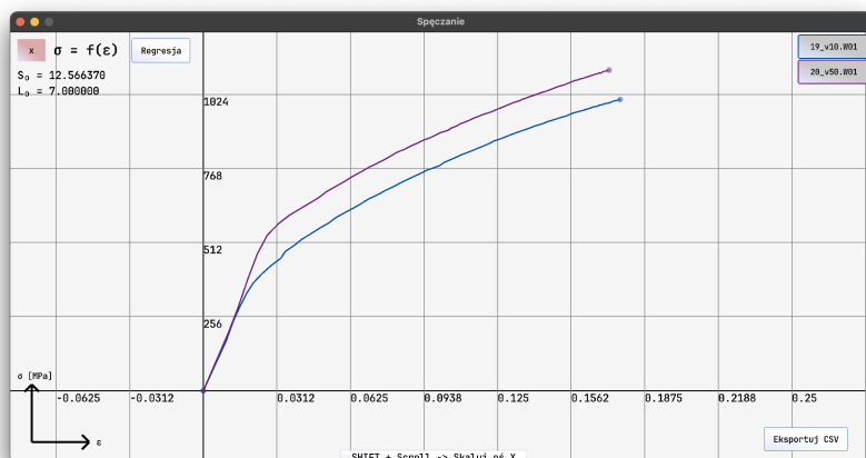
Rysunek 5.5: Wykres naprężenie-odkształcenie dla próbek BA1032 spęczanych w temperaturze otoczenia
