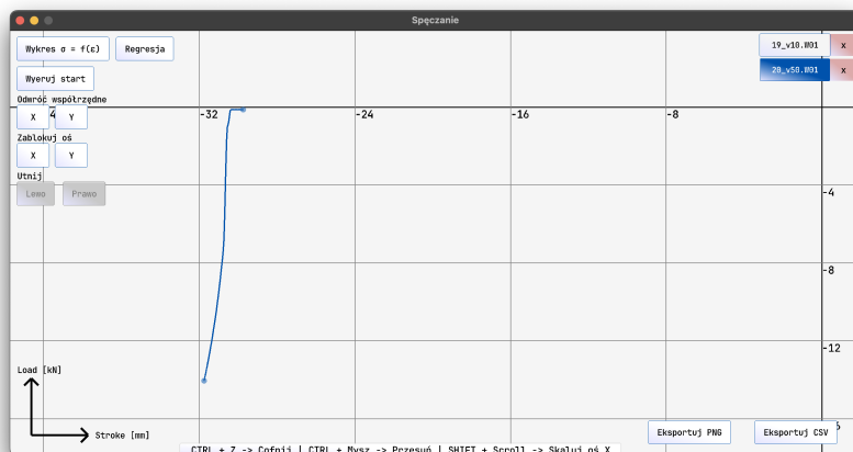
Rysunek 5.3: Wykres siły w funkcji przemieszczenia
