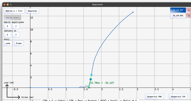
Rysunek 5.2: Wykres siły w funkcji przemieszczenia w trakcie operacji
