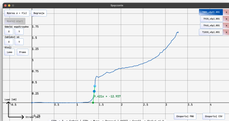
Rysunek 5.14: Wykres siły w funkcji przemieszczenia w trakcie operacji
