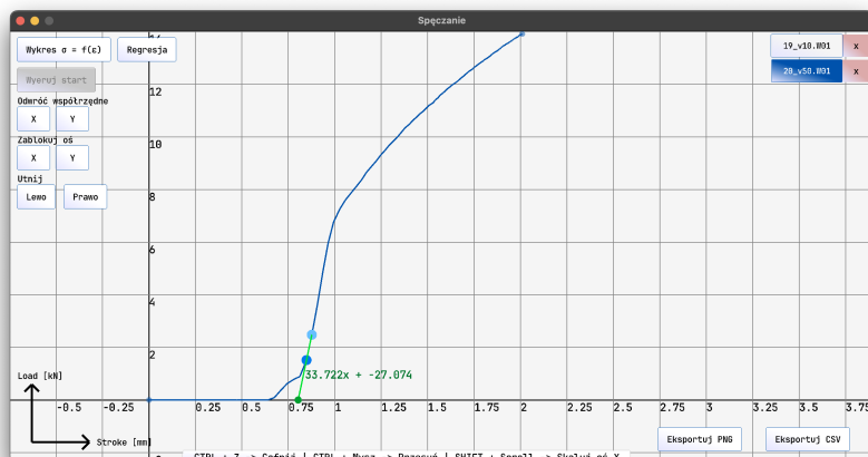
Rysunek 5.4: Wykres siły w funkcji przemieszczenia w trakcie operacji
