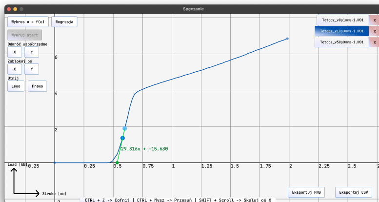
Rysunek 5.9: Wykres siły w funkcji przemieszczenia w trakcie operacji
