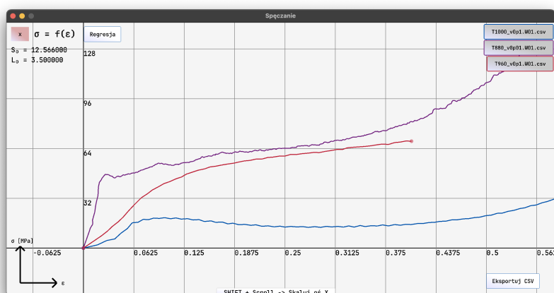
Rysunek 5.19: Wykres naprężenie-odkształcenie dla próbek CuSn6 spęczanych w stanie stałociękłym
