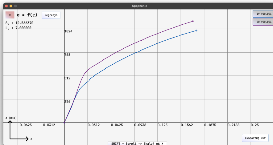
Rysunek 5.5: Wykres naprężenie-odkształcenie próbek 1 i 2
