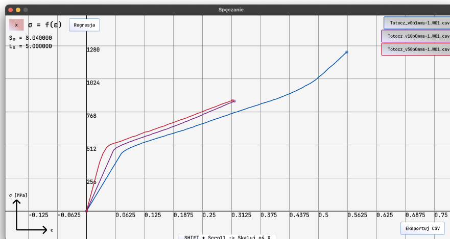
Rysunek 5.12: Wykres naprężenie-odkształcenie próbek 1, 2 i 3
