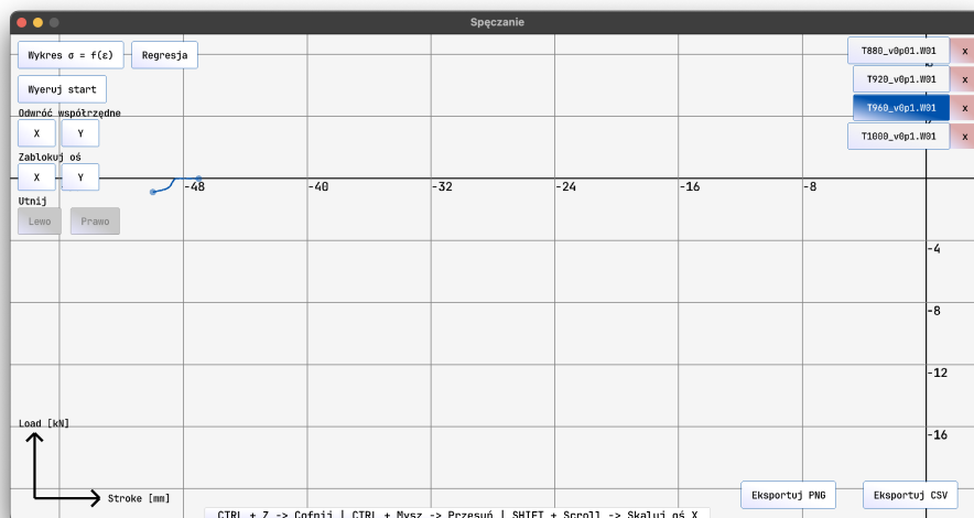
Rysunek 5.15: Wykres próbki 2 po zaimportowaniu
