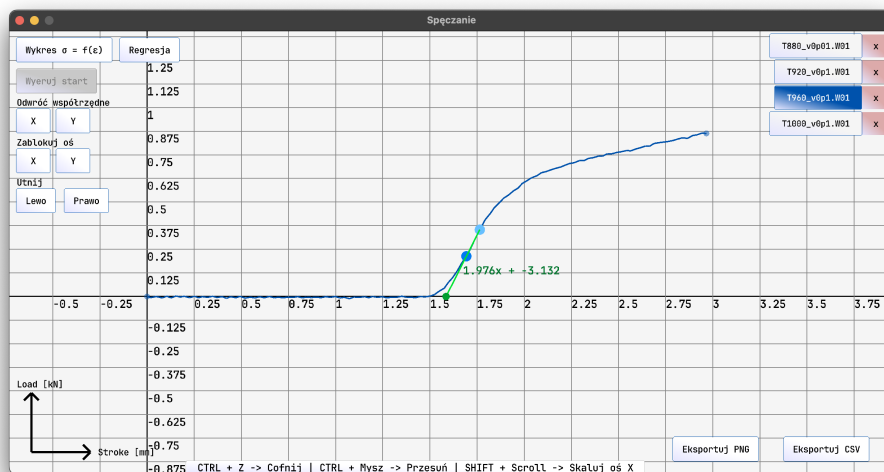
Rysunek 5.16: Wykres próbki 2 przy ekstrapolacji
