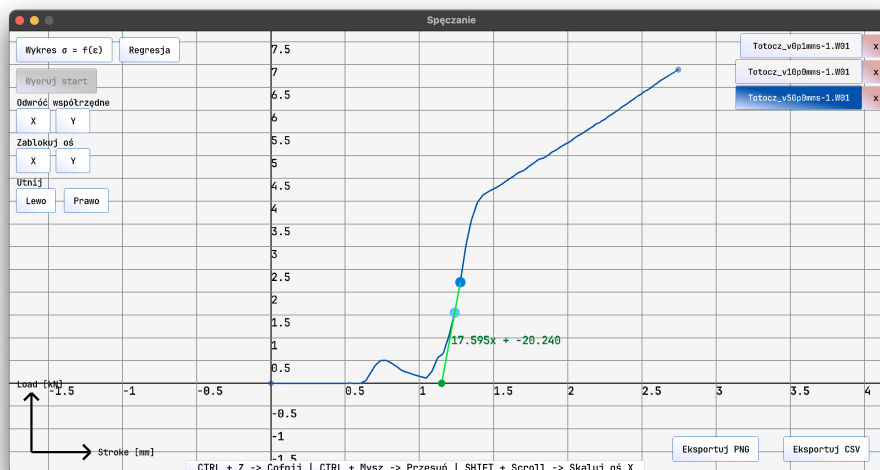
Rysunek 5.11: Wykres próbki 3 przy ekstrapolacji
