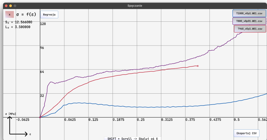
Rysunek 5.19: Wykres napężenie-odkształcenie próbek 1, 2 i 3
