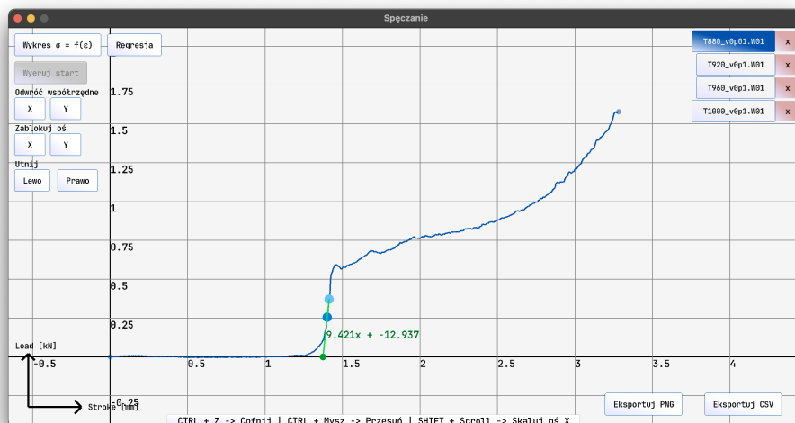
Rysunek 5.14: Wykres próbki 1 przy ekstrapolacji
