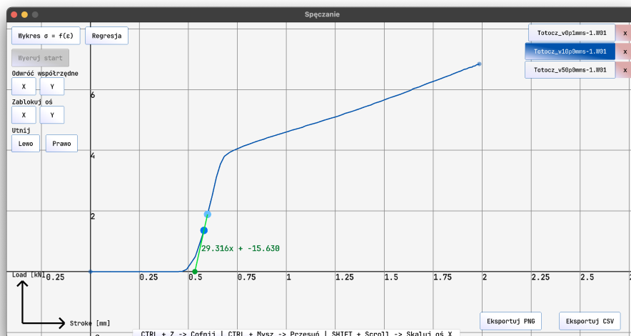
Rysunek 5.9: Wykres próbki 2 przy ekstrapolacji
