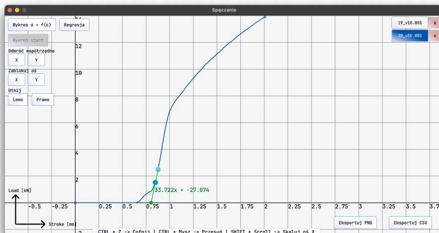
Rysunek 5.4: Wykres próbki 2 przy ekstrapolacji
