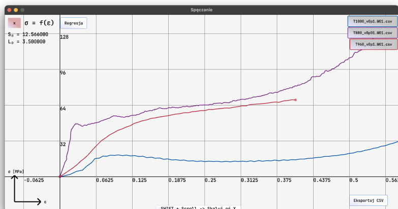
Rysunek 5.19: Wykres naprężenie-odkształcenie dla próbek CuSn6 spęczanych w stanie stałocięłym
