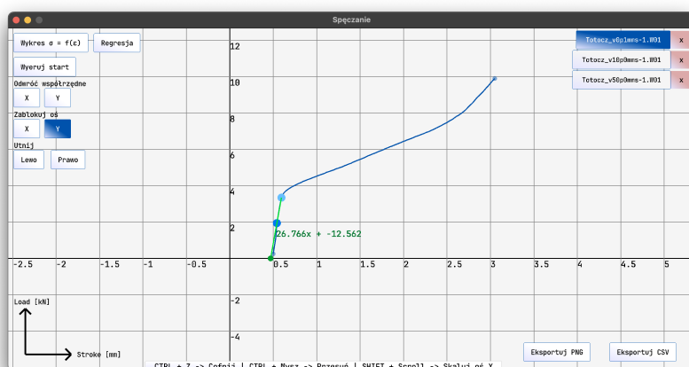
Rysunek 5.7: Wykres siły w funkcji przemieszczenia w trakcie operacji
