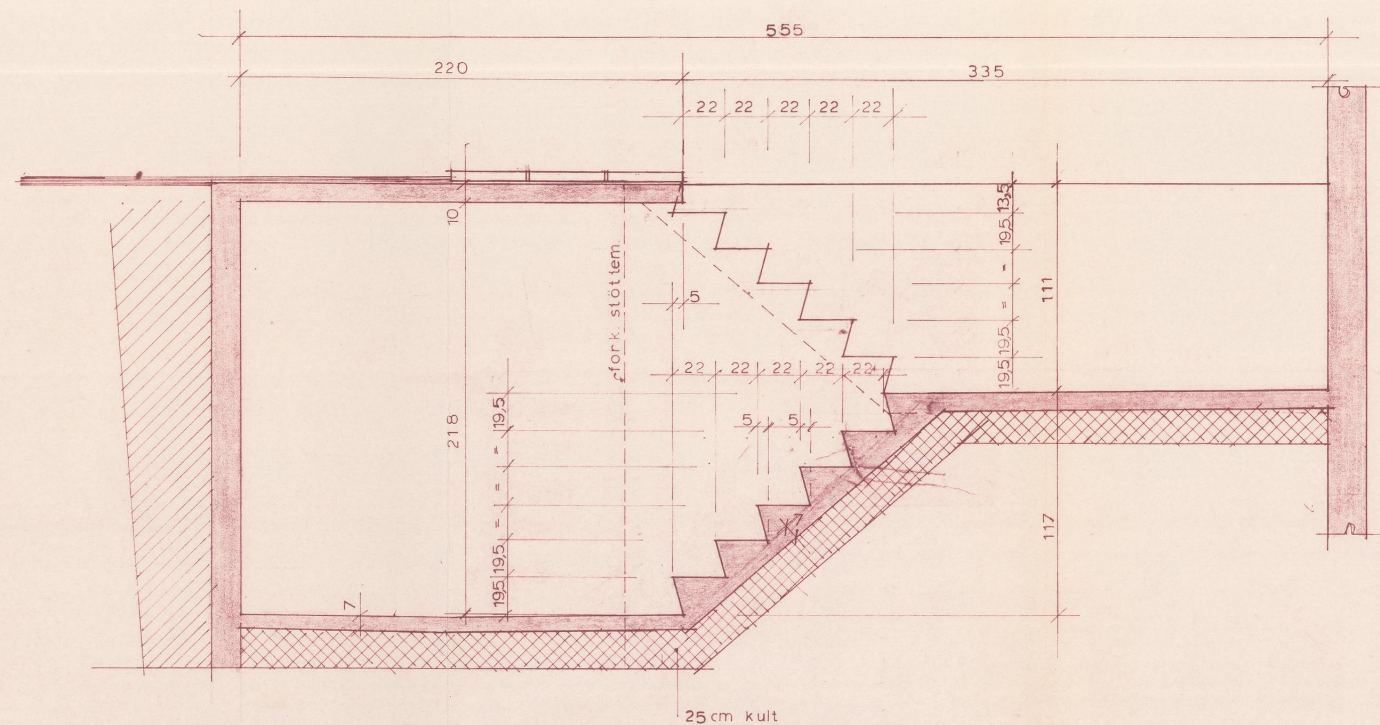
SNITT 5-5 M 1:20
