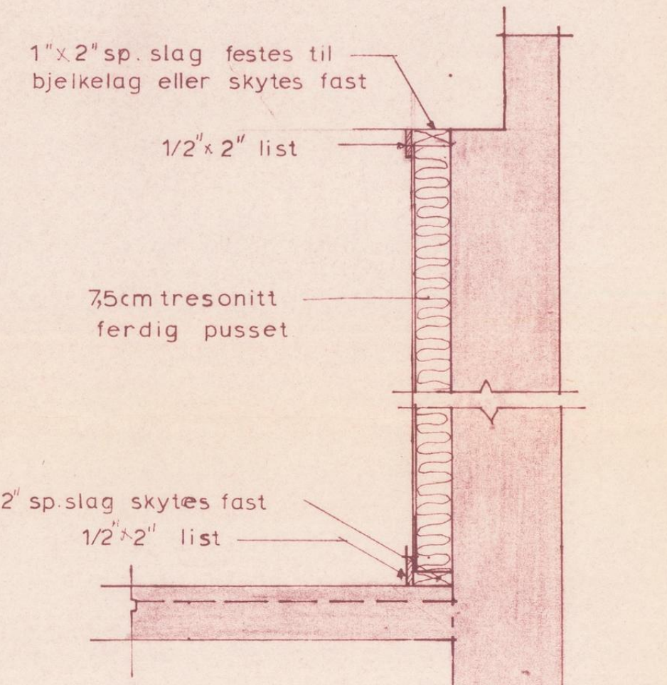
DETALJ F M 1:10
