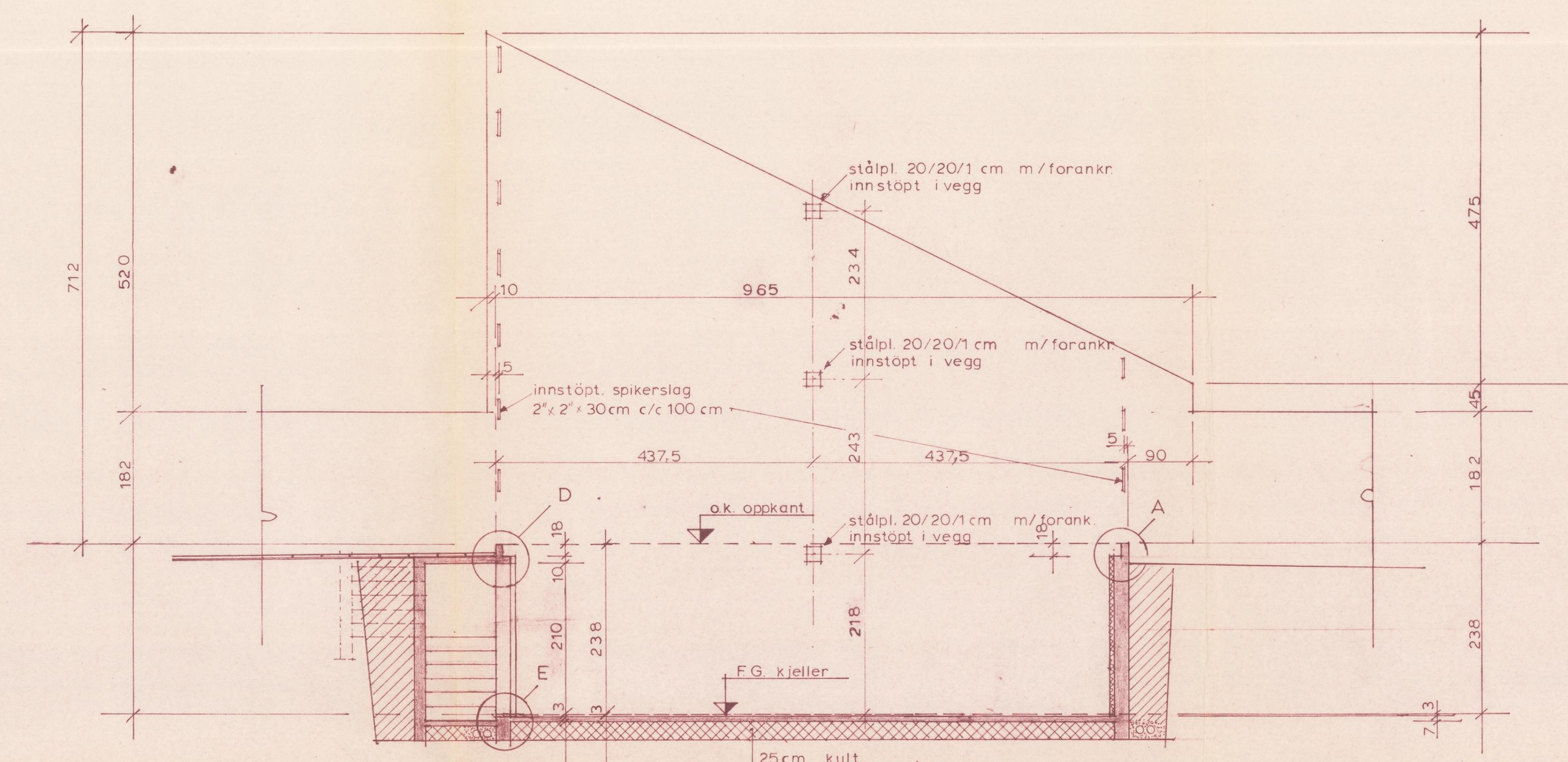
SNITT 2-2 M 1:50
