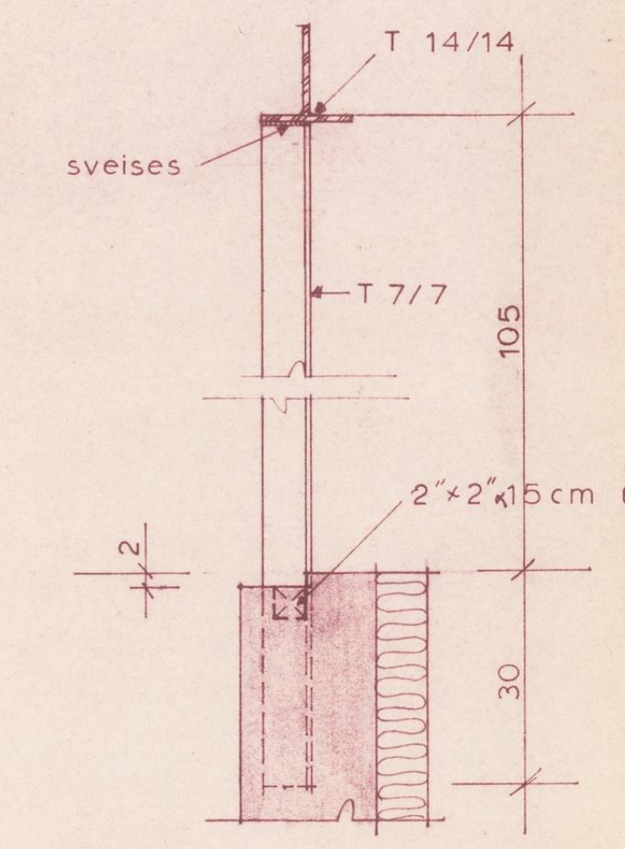
DETALJ B og C M 1:10
