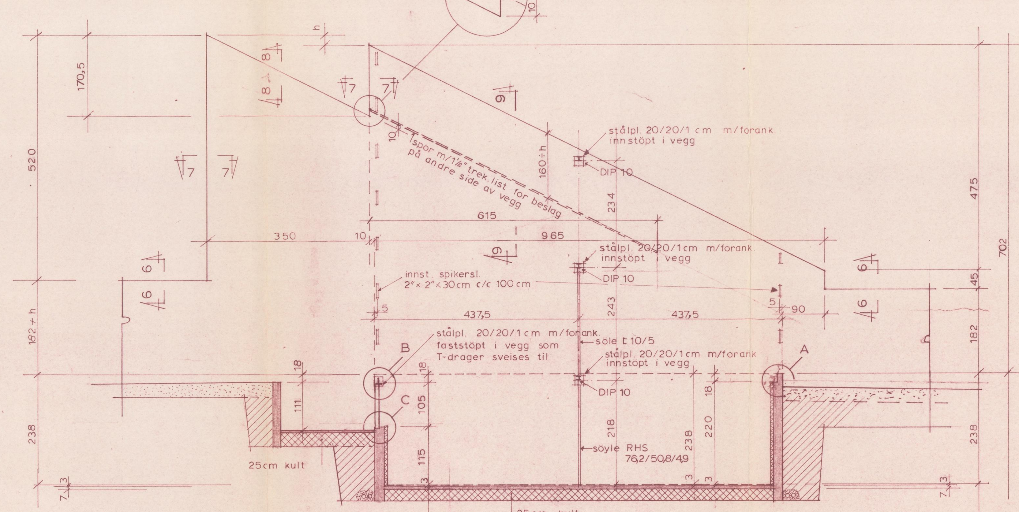
SNITT 1-1 M 1:50
