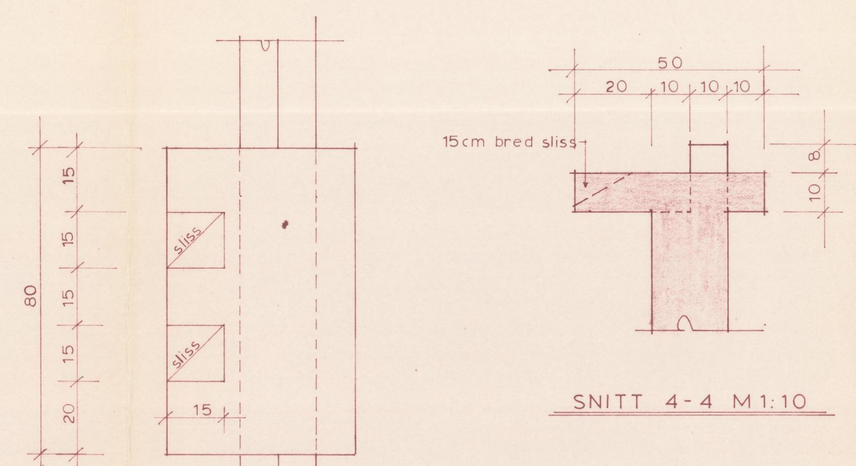
PLAN AV PIPEFUNDAMENT M 1:10
