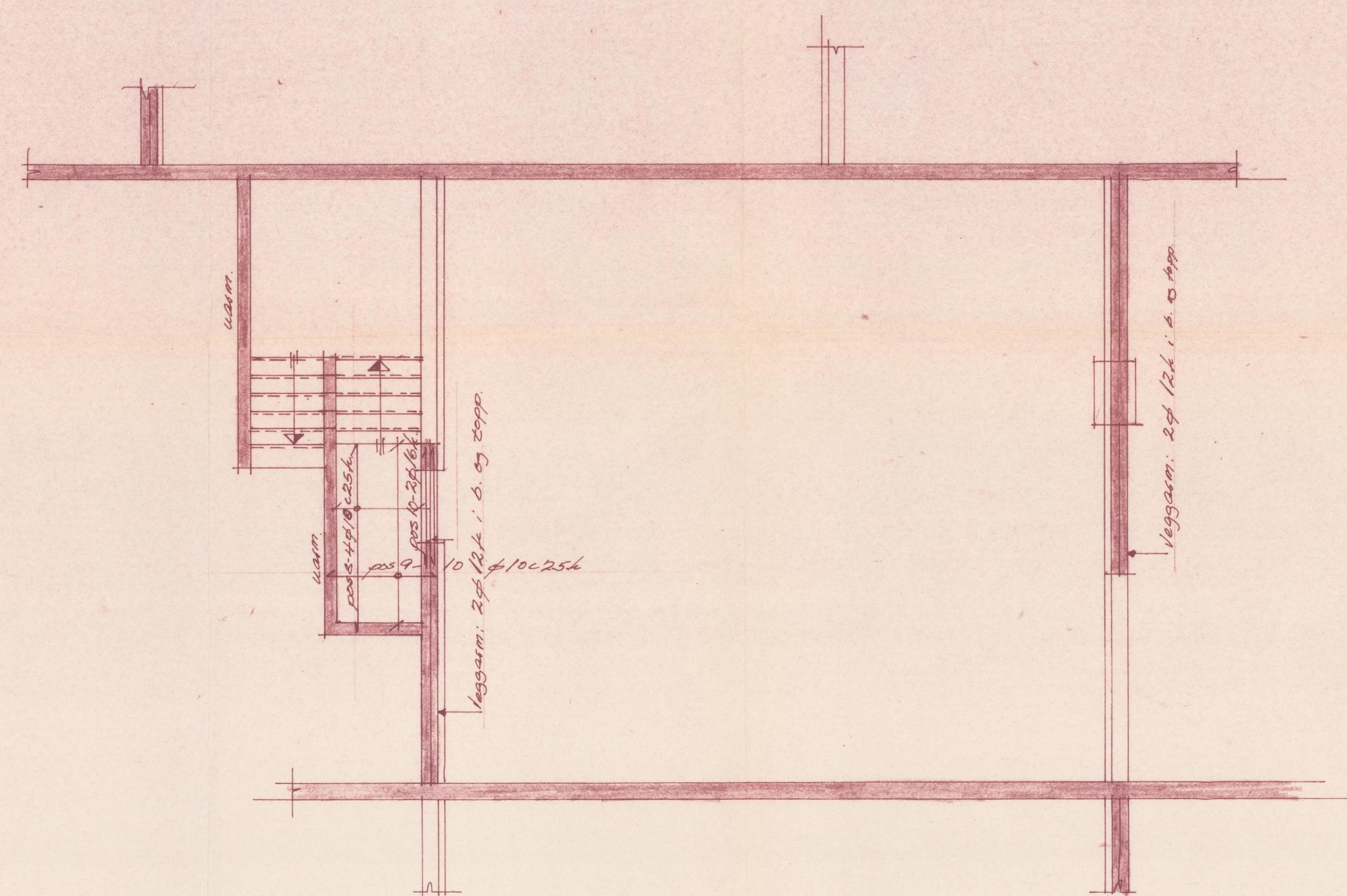
PLAN KJELLER M1:50
