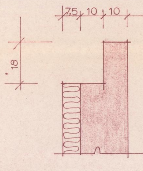
DETALJ A M 1:10
