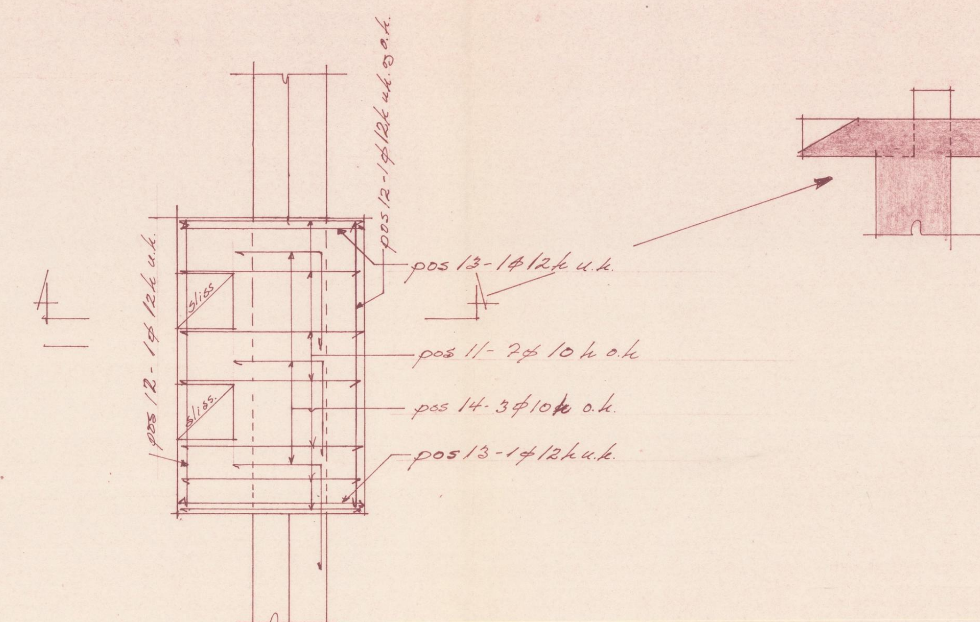
ARM. AV PEISFUNDAM. M1:10
