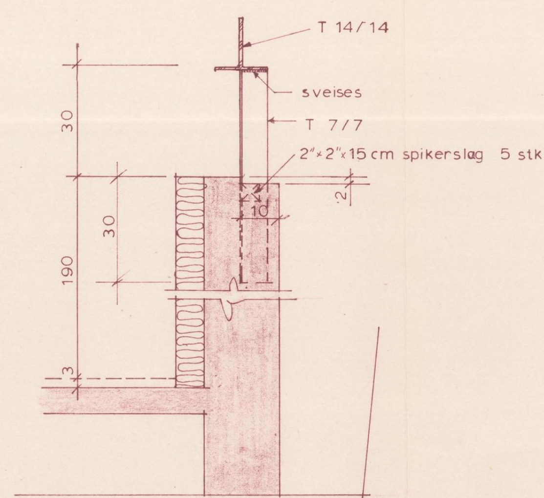
SNITT 3-3 M 1:10
