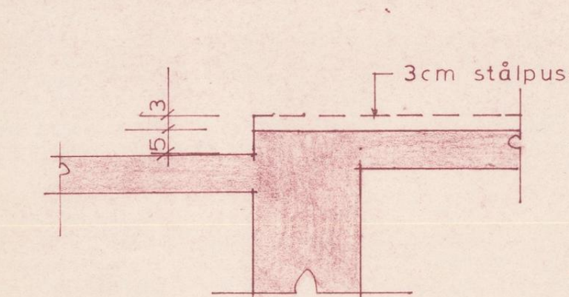
DETALJ E M 1:10
