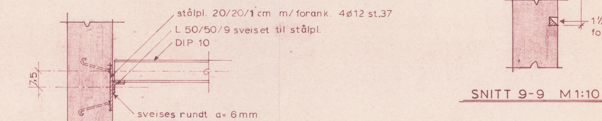
OPPLEGG AV STÅLDR M 1:10
