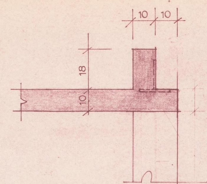
DETALJ D M 1:10
