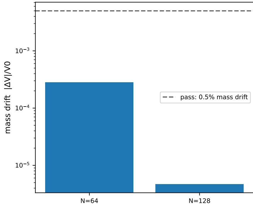
V10-a: mass drift (Olsson--Kreiss corr.)
