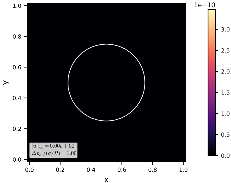
A: \alpha=1 , nominal \epsilon
