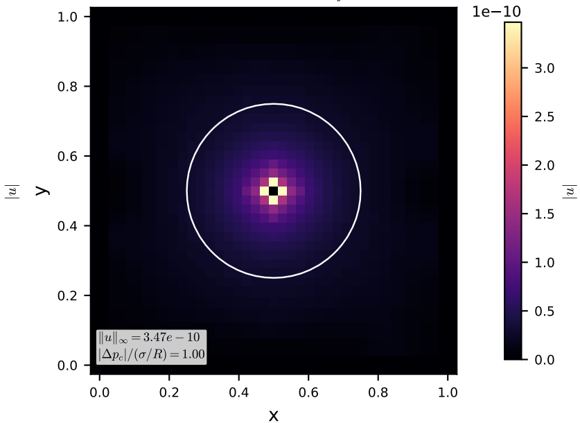
C: \alpha=2 , local \epsilon_{ij}
