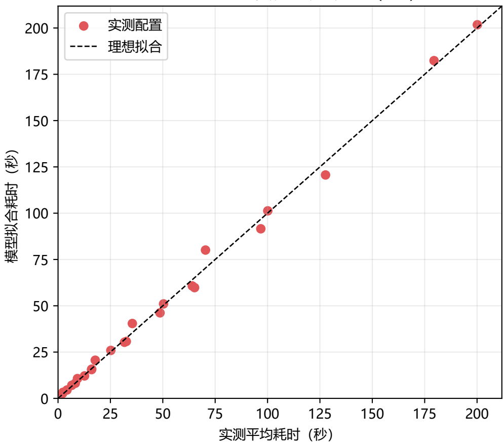
Paillier 总耗时的实测--拟合关系 (M4)
