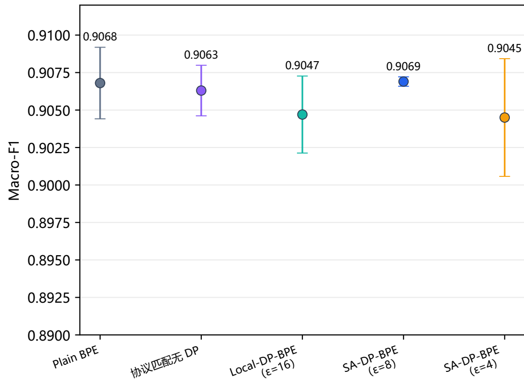
AG News 下游效用
