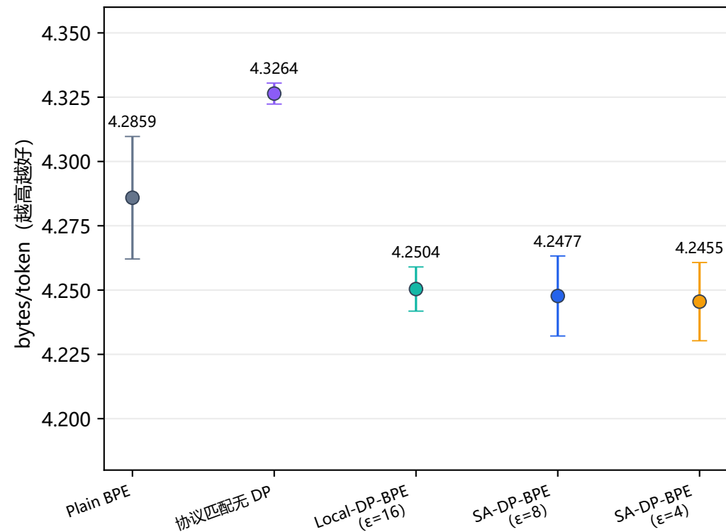
留出 C4 编码效率
