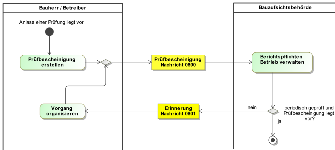
Abbildung III.19.2. Prozess Überwachungspflichtige Anlagen
