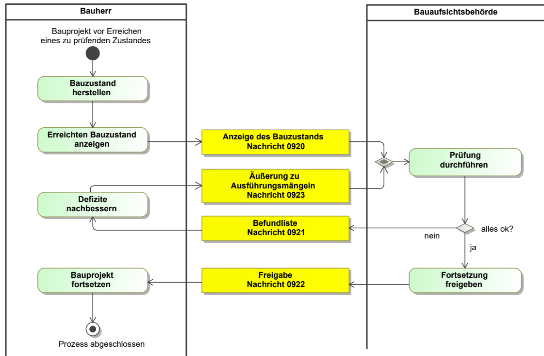
Abbildung III.18.2. Prozess Anzeige Bauzustand
