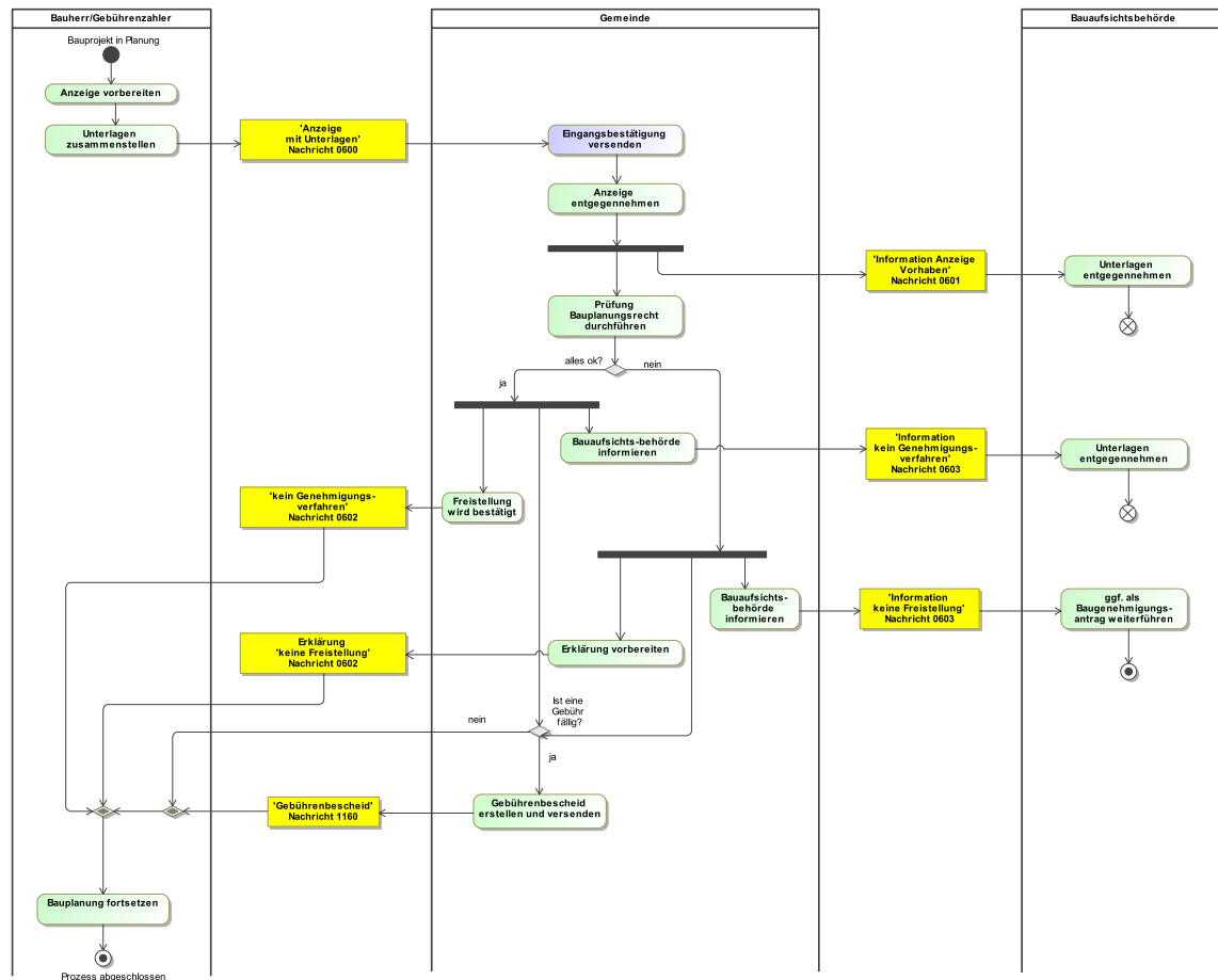
Abbildung III.8.2. Prozess Prüfung Genehmigungsfreistellung
