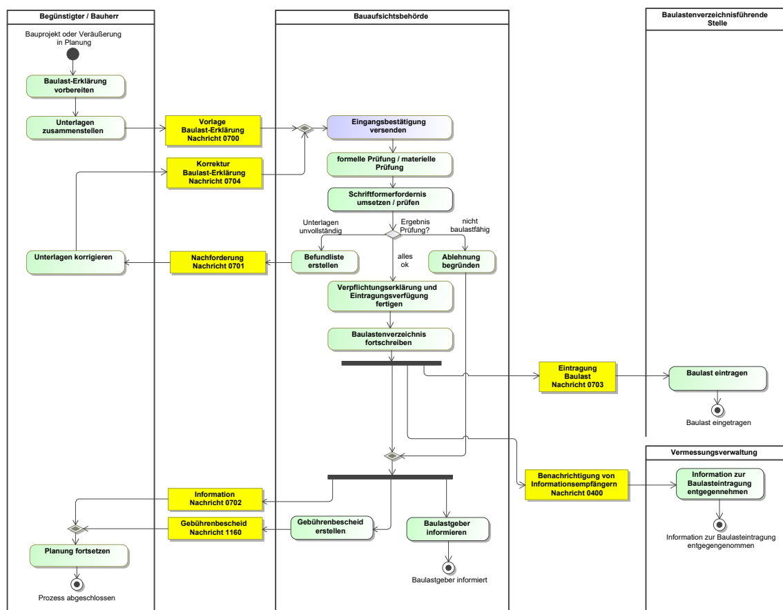
Abbildung III.16.2. Prozess Eintragung Baulast
