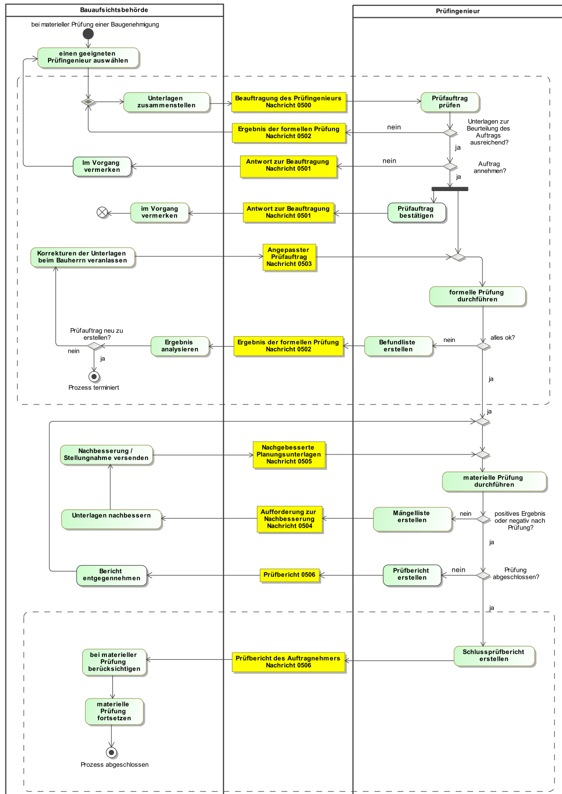
Abbildung III.13.2. Prozess Bautechnische Nachweise prüfen (Bauaufsichtsbehörde)
