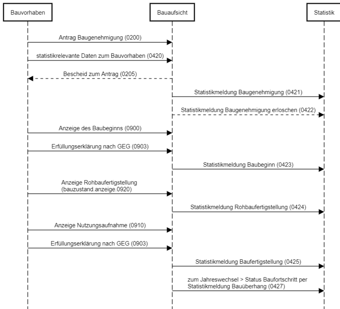
Abbildung III.12.4. Nachrichtensequenz und Übermittlungsanlässe
