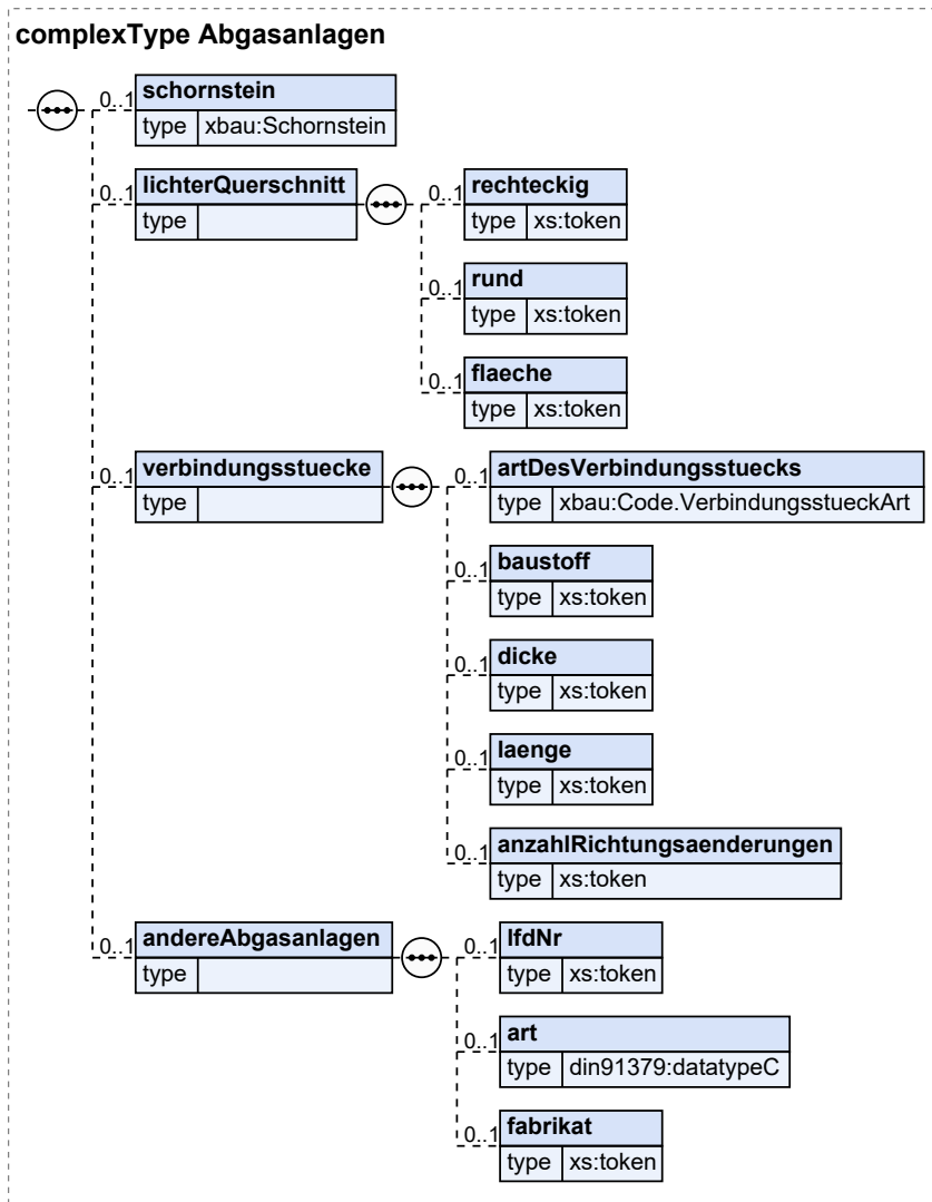
Abbildung II.4.71. Abgasanlagen
