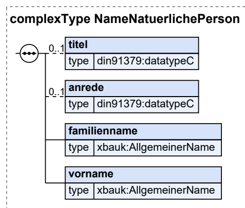
Abbildung III.2.4. NameNatuerlichePerson
