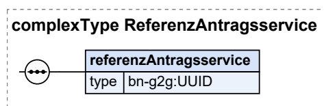
Abbildung III.5.7. ReferenzAntragsservice
