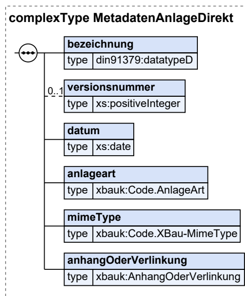
Abbildung III.4.3. MetadatenAnlageDirekt
