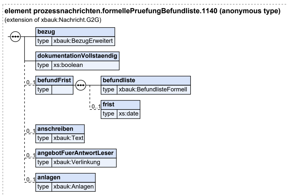
Abbildung III.8.16. prozessnachrichten.formellePruefungBefundliste.1140
