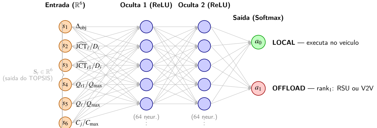
Figura 17 – Arquitetura da rede Actor (MLP 6 → 64 → 64 → 2): o vetor de estado compacto S_t produzido pelo TOPSIS alimenta duas camadas ocultas com ativação ReLU; a camada Softmax final emite as probabilidades das ações a_0 (LOCAL) e a_1 (OFFLOAD rank_1 ).
