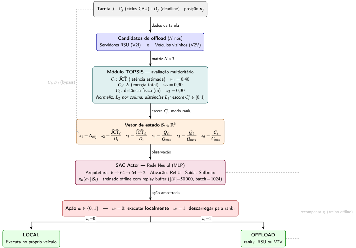
Figura 16 – Arquitetura SAC-TOPSIS: fluxo vertical de decisão. O módulo TOPSIS comprime N candidatos em vetor fixo \mathbb{R}^6 ; o SAC Actor decide binariamente entre execução local e offload para o rank_1 . A seta tracejada cinza indica bypass direto de C_j e D_j ; a tracejada direita mostra o loop de recompensa durante o treinamento offline .
