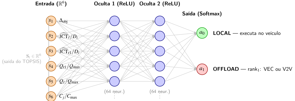
Figura 17 – Arquitetura da rede Actor (MLP 6 \rightarrow 64 \rightarrow 64 \rightarrow 2 ): o vetor de estado compacto \mathbf{S}_t produzido pelo TOPSIS alimenta duas camadas ocultas com ativação ReLU; a camada Softmax final emite as probabilidades das ações a_0 (LOCAL) e a_1 (OFFLOAD rank_1 ).
