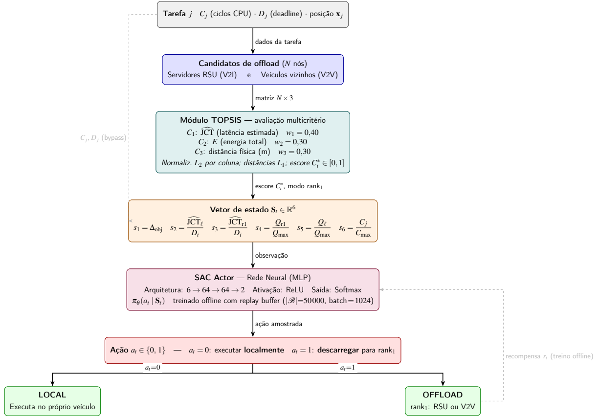
Figura 17 – Arquitetura SAC-TOPSIS: fluxo vertical de decisão. O módulo TOPSIS comprime N candidatos em vetor fixo \mathbb{R}^6 ; o SAC Actor decide binariamente entre execução local e offload para o \text{rank}_1 . A seta tracejada cinza indica bypass direto de C_j e D_j ; a tracejada direita mostra o loop de recompensa durante o treinamento offline .
