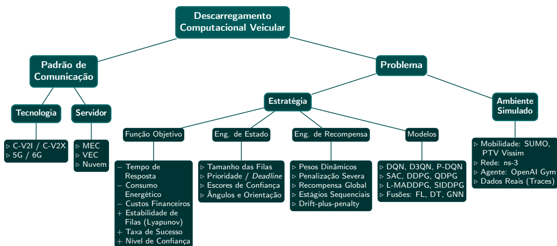
Figura 15 – Taxonomia adaptada para classificação dos trabalhos relacionados em descarregamento computacional veicular, com ênfase na modelagem de Aprendizado por Reforço Profundo (DRL) e ambiente de simulação.
