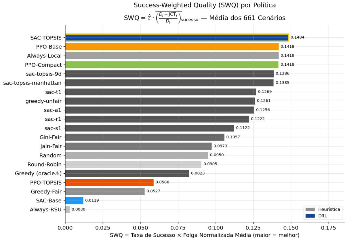
Figura 19 – SWQ médio por política sobre 661 cenários de teste ( \alpha = 0,35 , \beta = 0,35 , \gamma = 0,30 ). Barras em cinza representam heurísticas; barras escuras representam políticas DRL. A borda dourada indica a melhor política. Maior é melhor.
