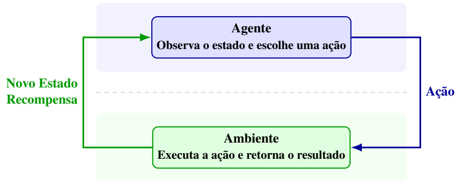
Figura 10 – Ciclo básico de interação Agente-Ambiente no RL. A cada passo, o agente observa o estado atual, escolhe uma ação, e o ambiente responde com uma recompensa e um novo estado.
