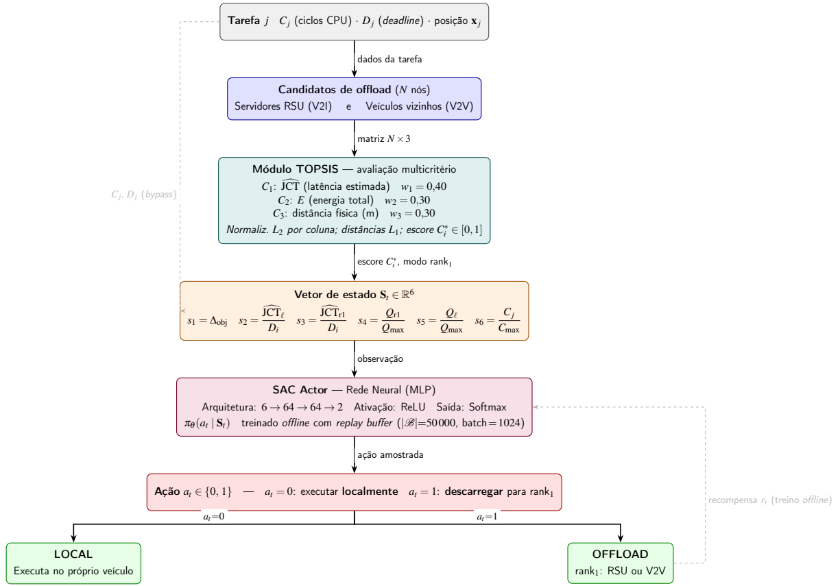
Figura 15 – Arquitetura SAC-TOPSIS: fluxo vertical de decisão. O módulo TOPSIS comprime N candidatos em vetor fixo \mathbb{R}^6 ; o SAC Actor decide binariamente entre execução local e offload para o rank_1 . A seta tracejada cinza indica bypass direto de C_j e D_j ; a tracejada direita mostra o loop de recompensa durante o treinamento offline.
