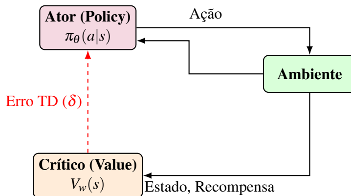
Figura 12 – Dinâmica Ator-Crítico.
