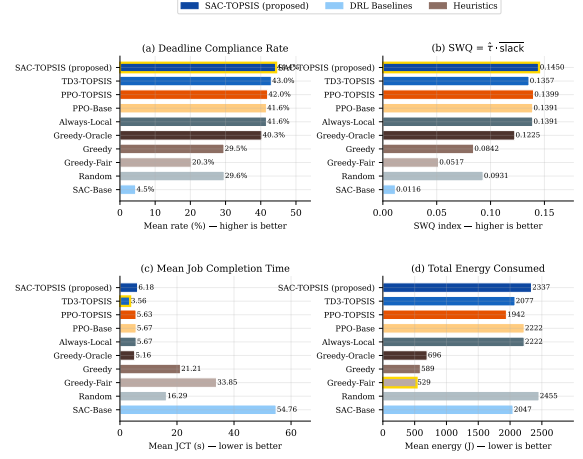
Figura 2 Comparação de desempenho entre as principais métricas. O SAC-TOPSIS (azul escuro) alcança a maior taxa de cumprimento de prazo e o maior índice SWQ. A borda dourada marca o melhor valor em cada gráfico.
