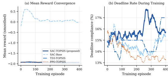
Figura 5 Convergência do treinamento ao longo de 400 episódios. (a) Recompensa média (suavizada com janela de 20 episódios); (b) taxa de cumprimento de prazo durante o treinamento. O SAC-TOPSIS alcança convergência estável em ambas as métricas.
