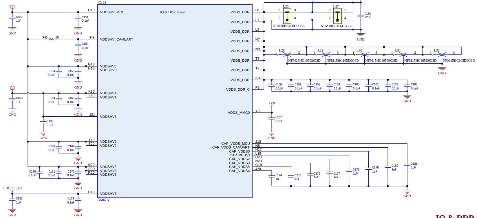
IO & DDR Power
