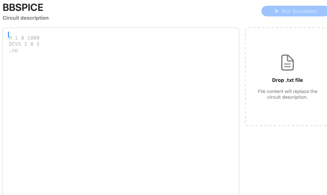
Rysunek 4.1: Główne okno aplikacji z edytorem opisu układu
