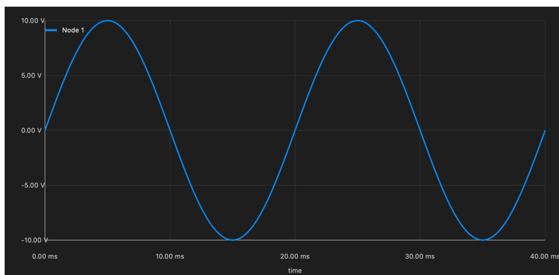
Rysunek 4.1: Wynik analizy czasowej prostego układu ze źródłem sinusoidalnym i rezystorem
