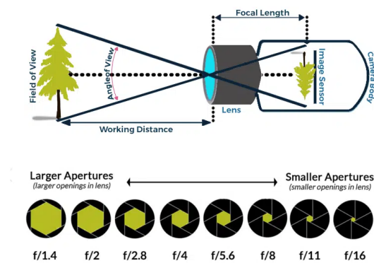
Abbildung 3: Schematische Darstellung einer Linse mit den wichtigsten Parametern. 78
