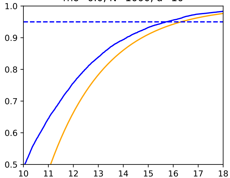
\rho=0.0, N=1000, d=10
