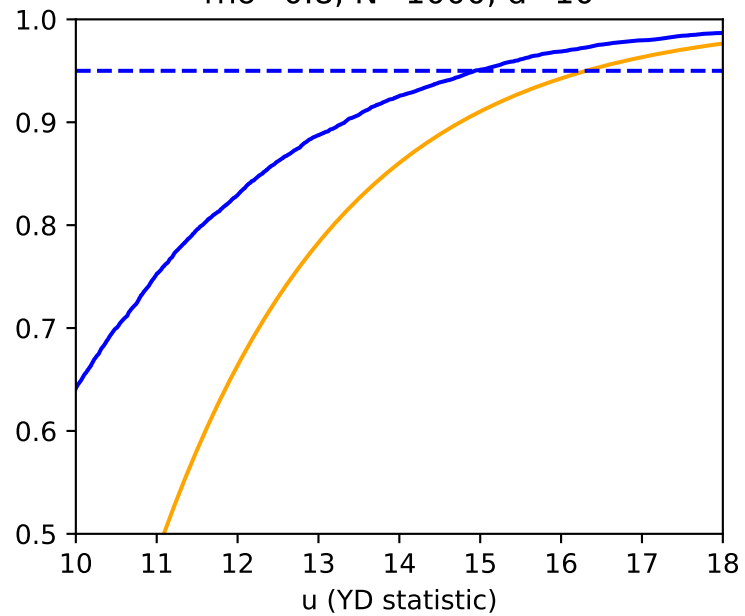
\rho=0.8, N=1000, d=10
