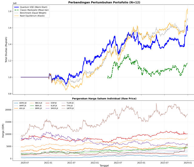
Gambar: Perbandingan Pertumbuhan Modal Strategi VQE terhadap Tolok Ukur Klasik (N=12)
