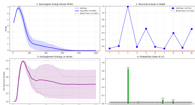
Analisis VQE tanpa Warm-Start - Jendela 2022-07-22 (N=6, K=3)
