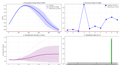
Analisis VQE tanpa Warm-Start - Jendela 2022-06-23 (N=6, K=3)
