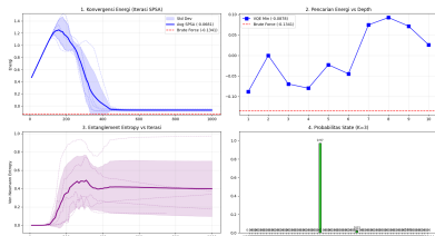
Analisis VQE Warm-Start - Jendela 2022-07-22 (N=6, K=3)
