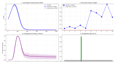
Analisis VQE Warm-Start - Jendela 2023-03-17 (N=6, K=3)
