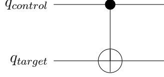
Gambar 2.10: Representasi simbolik gerbang keterbelitan CNOT yang mengilustrasikan interaksi non-lokal antar qubit dalam sistem sirkuit.
