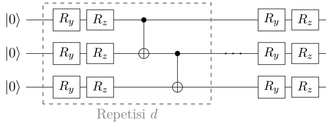
Gambar 2.5: Visualisasi arsitektur sirkuit kuantum EfficientSU2 dengan lapisan rotasi parameterisasi dan keterbelitan berantai ( linear connectivity ).
