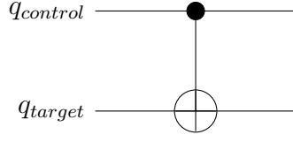
Gambar 2.13: Representasi simbolik gerbang keterbelitan ( Controlled-NOT ) yang mengilustrasikan interaksi non-lokal antar qubit dalam sistem sirkuit.
