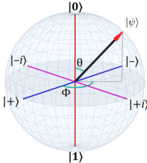
Gambar 2.7: Representasi Bola Bloch sebagai visualisasi geometris keadaan murni sebuah qubit . Posisi vektor keadaan ditentukan oleh sudut polar \theta dan sudut azimutal \phi , yang dipetakan ke koordinat Kartesian (x, y, z) .
