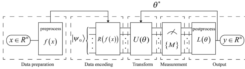
Gambar 2.14: Representasi alur kerja sirkuit kuantum berparameter (PQC) yang mengilustrasikan tahap penyandian data, sirkuit variasional, pengukuran, dan pembaruan parameter oleh algoritma optimasi klasik.
