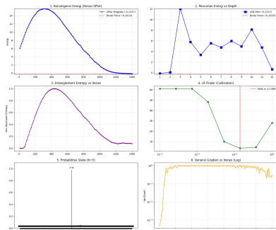
Analisis VQE Warm-Start - Jendela 2023-02-16 (N=10, K=5)
