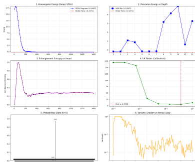
Analisis VQE tanpa Warm-Start - Jendela 2021-11-10 (N=10, K=5)
