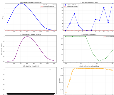
Analisis VQE Warm-Start - Jendela 2022-03-14 (N=10, K=5)
