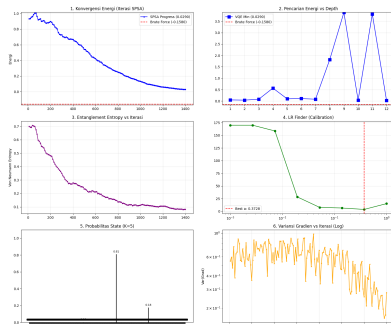
Analisis VQE tanpa Warm-Start - Jendela 2021-08-10 (N=10, K=5)
