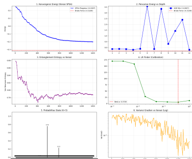
Analisis VQE tanpa Warm-Start - Jendela 2021-10-11 (N=10, K=5)
