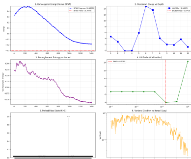
Analisis VQE Warm-Start - Jendela 2022-04-12 (N=10, K=5)
