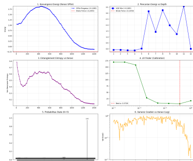
Analisis VQE tanpa Warm-Start - Jendela 2022-12-19 (N=10, K=5)
