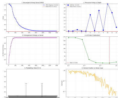
Analisis VQE tanpa Warm-Start - Jendela 2021-02-02 (N=10, K=5)
