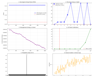
Analisis VQE Warm-Start - Jendela 2021-02-02 (N=10, K=5)
