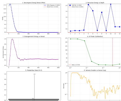
Analisis VQE tanpa Warm-Start - Jendela 2022-04-12 (N=10, K=5)
