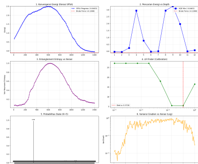
Analisis VQE Warm-Start - Jendela 2023-05-30 (N=10, K=5)
