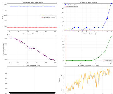
Analisis VQE Warm-Start - Jendela 2022-12-19 (N=10, K=5)
