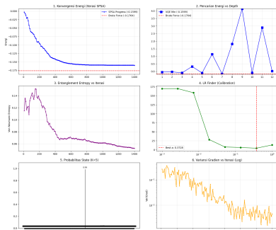
Analisis VQE tanpa Warm-Start - Jendela 2023-10-05 (N=10, K=5)
