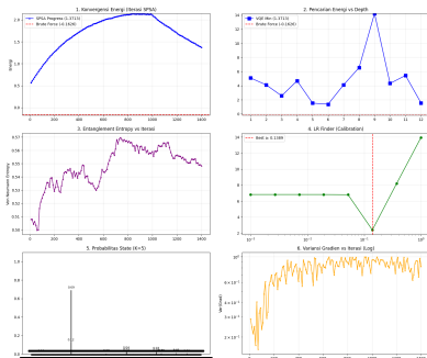
Analisis VQE Warm-Start - Jendela 2021-09-10 (N=10, K=5)
