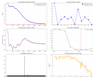
Analisis VQE tanpa Warm-Start - Jendela 2023-07-05 (N=10, K=5)
