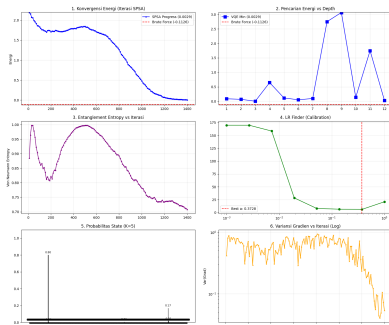
Analisis VQE tanpa Warm-Start - Jendela 2023-03-17 (N=10, K=5)
