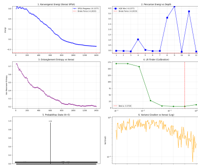
Analisis VQE tanpa Warm-Start - Jendela 2023-02-16 (N=10, K=5)
