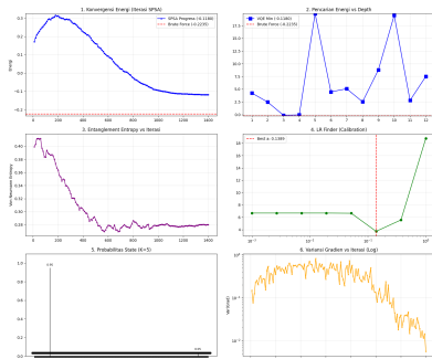
Analisis VQE Warm-Start - Jendela 2021-12-09 (N=10, K=5)
