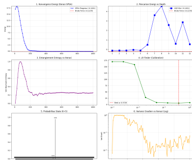
Analisis VQE tanpa Warm-Start - Jendela 2021-12-09 (N=10, K=5)
