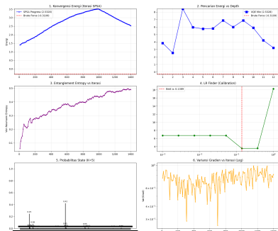
Analisis VQE Warm-Start - Jendela 2021-10-11 (N=10, K=5)
