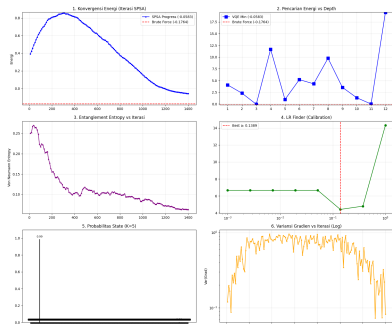
Analisis VQE Warm-Start - Jendela 2023-10-05 (N=10, K=5)
