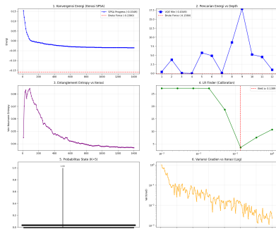
Analisis VQE Warm-Start - Jendela 2021-08-10 (N=10, K=5)
