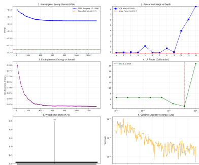
Analisis VQE Warm-Start - Jendela 2023-08-04 (N=10, K=5)
