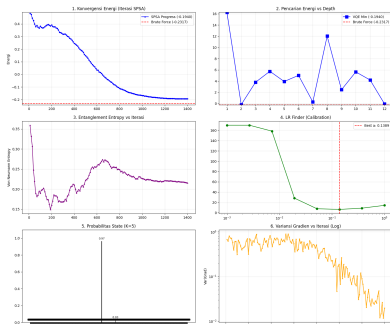
Analisis VQE tanpa Warm-Start - Jendela 2023-08-04 (N=10, K=5)
