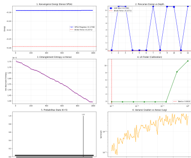
Analisis VQE Warm-Start - Jendela 2021-11-10 (N=10, K=5)
