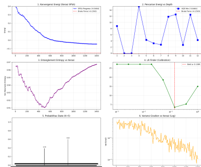
Analisis VQE Warm-Start - Jendela 2023-07-05 (N=10, K=5)
