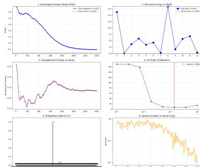
Analisis VQE tanpa Warm-Start - Jendela 2021-09-10 (N=10, K=5)
