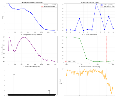
Analisis VQE tanpa Warm-Start - Jendela 2023-05-30 (N=10, K=5)
