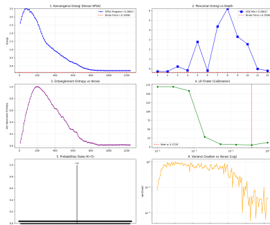
Analisis VQE tanpa Warm-Start - Jendela 2022-03-14 (N=10, K=5)
