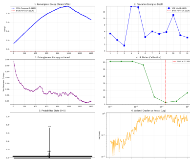
Analisis VQE Warm-Start - Jendela 2023-03-17 (N=10, K=5)
