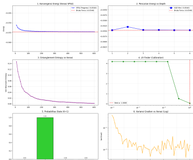
Analisis VQE tanpa Warm-Start - Jendela 2021-08-10 (N=2, K=1)
