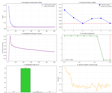
Analisis VQE Warm-Start - Jendela 2021-07-09 (N=2, K=1)
