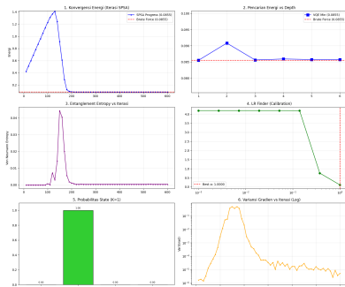
Analisis VQE tanpa Warm-Start - Jendela 2021-07-09 (N=2, K=1)
