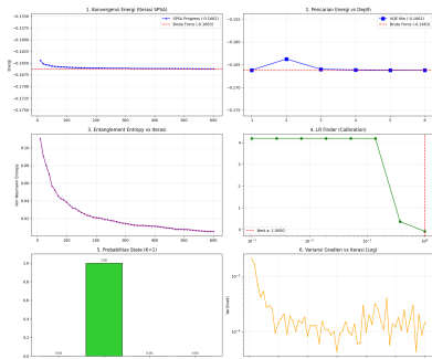
Analisis VQE tanpa Warm-Start - Jendela 2021-03-04 (N=2, K=1)
