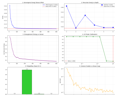
Analisis VQE Warm-Start - Jendela 2021-03-04 (N=2, K=1)
