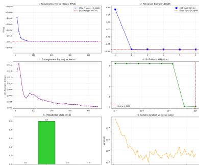
Analisis VQE Warm-Start - Jendela 2021-08-10 (N=2, K=1)
