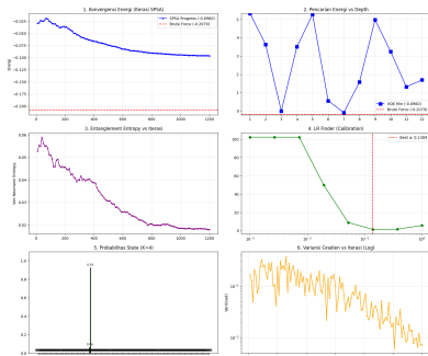
Analisis VQE tanpa Warm-Start · jendela 2021-02-02 (N=8, K=4)
