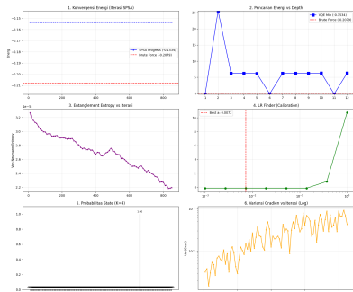
Analisis VQE Warm-Start · jendela 2021-02-02 (N=8, K=4)
