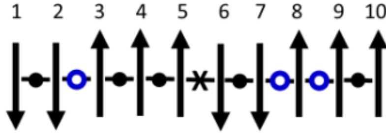
Gambar 2.6: Representasi visual model Ising satu dimensi (1D) yang menunjukkan dinamika orientasi spin dan klasifikasi energi interaksi ( \bullet , \times , \circ ) di bawah pengaruh fluktuasi termal (Chamberlin & Lindsay, 2024).
