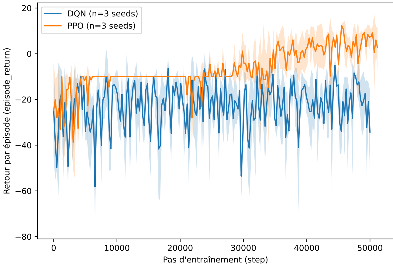
Courbes d'apprentissage - moyenne \pm écart-type sur les seeds
