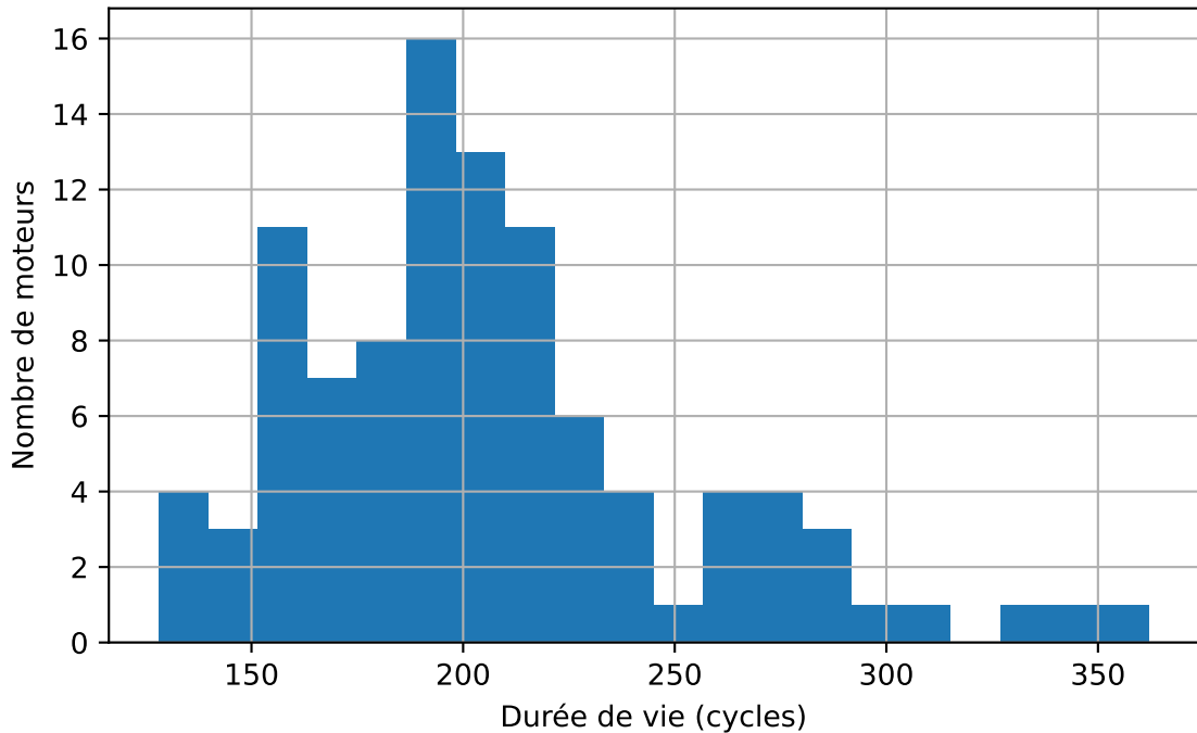
Distribution des durées de vie - FD001 train
