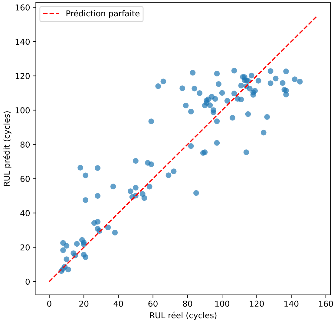
RUL prédit vs réel - Random Forest (RMSE=18.2)
