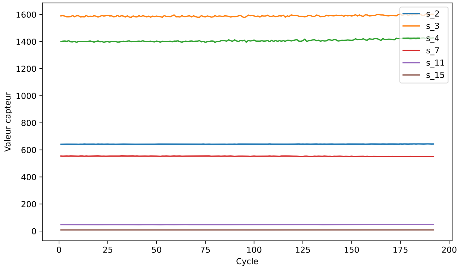
Trajectoire de dégradation - moteur 1 (FD001)
