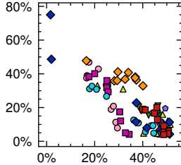
ilmageNet-R200/10
