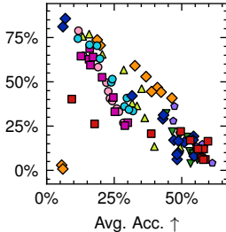
iCRe50/10
