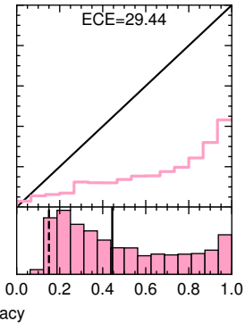
LoRA
