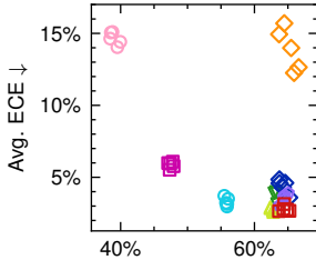
iCIFAR100/10
