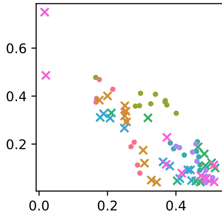
ilmageNet-R200/10
