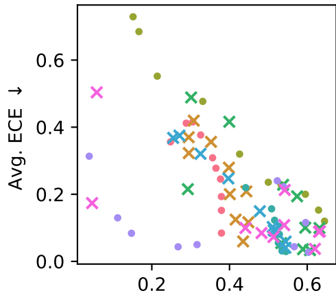
iCIFAR100/10
