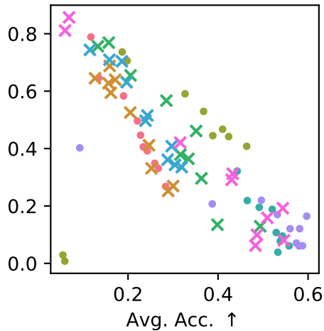
iCOPRe50/10
