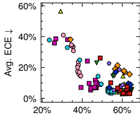
iCIFAR100/10
