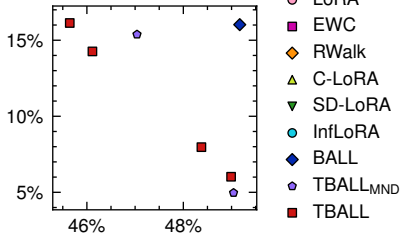
ilmageNet-R200/10
