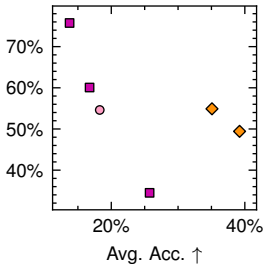
iCOnRe50/10
