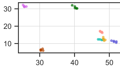
ilmageNet-R200/10
