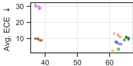
iCIFAR100/10
