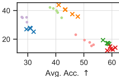
iCore50/10
