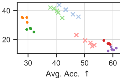
iCore50/10
