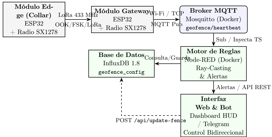
Figura 1: Topología general del sistema de geofencing ganadero y flujo de información entre capas.
