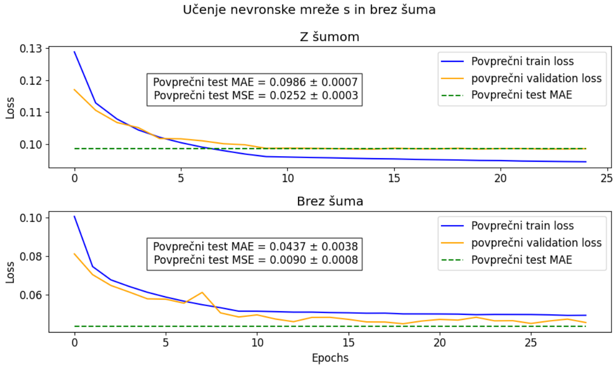
Slika 7: Povprečne funkcije izgube nevronske mreže, ki smo jo učili na zašumljenih ter nezašumljenih podatkih. Prikazani sta funkcija izgube validacijske množice ter trening množice. Prav tako je s črtkano zeleno črto prikazano MAE odstopanje med napovedjo mreže ter testnimi podatki.
