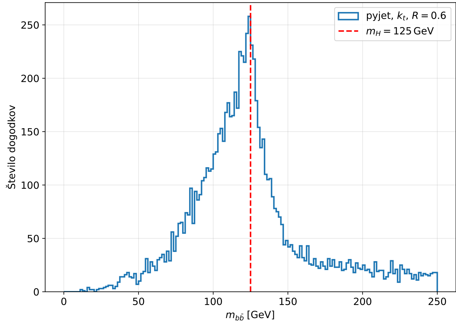
Spekter rekonstruiranih invariantnih mas
