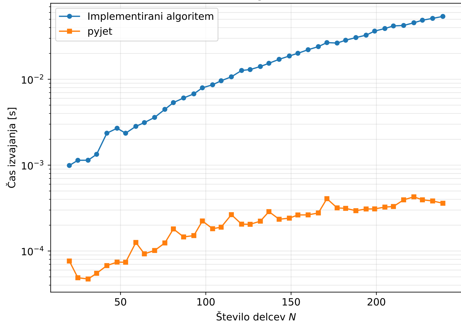
Časovna zahtevnost algoritmov za k_t , R = 0.6
