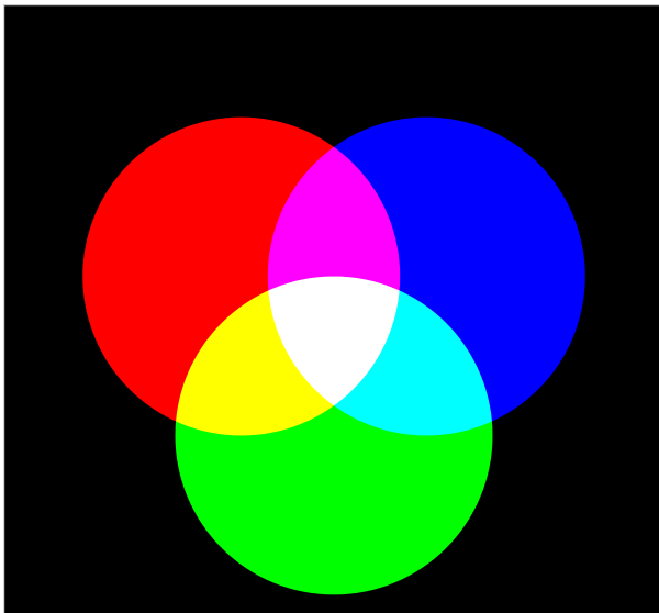
光の三原色 (加法混色)
