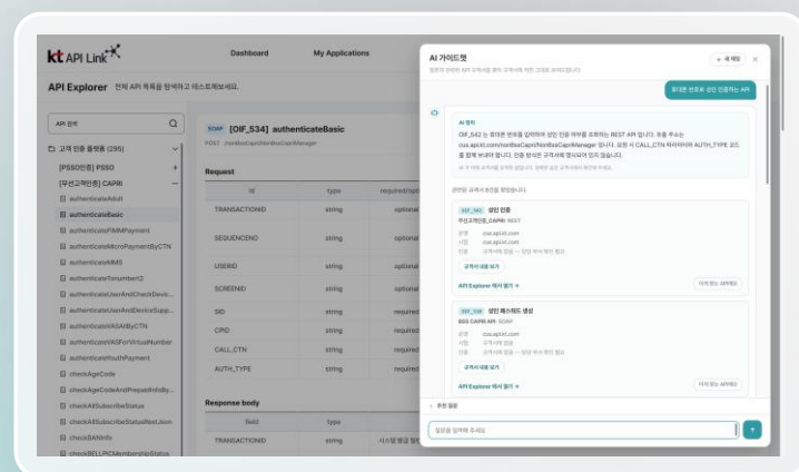
AI 가이드챗 자연어 질문과 원문 근거
