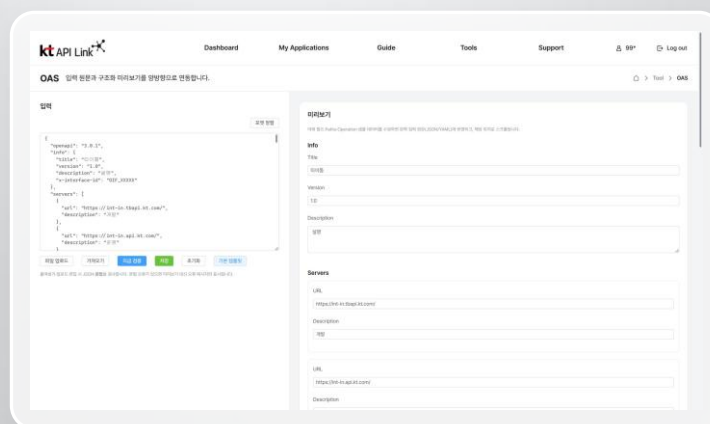
OAS 명세 도구 OpenAPI 명세 작성 · 미리보기
