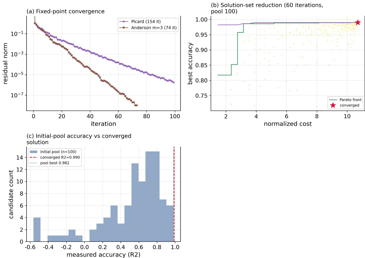
그림 4. 해공간 탐색과 수렴 거동. (a) 가속 기법과 an iterative solver 반복의 잔차 수렴 비교; (b) 해집합 축소 반복의 후보군-비지배 전선과 최고 정확도 수렴 궤적; (c) 초기 후보 풀(전수 실행) 정확도 분포와 수렴 차기 해의 개선포.
